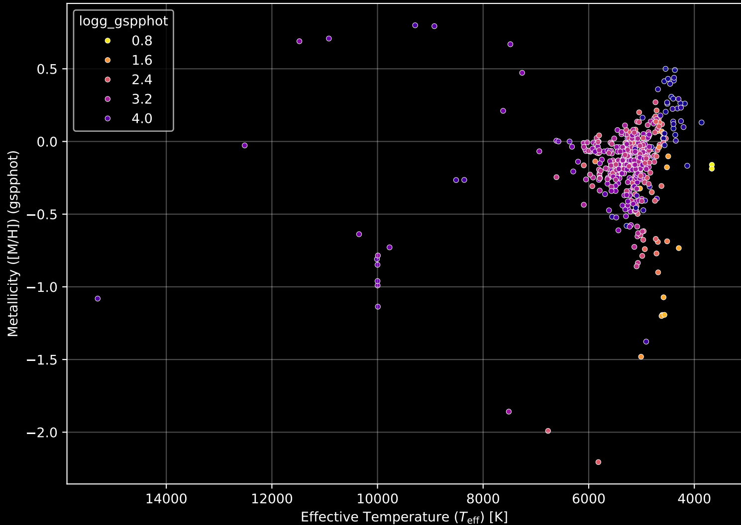
APOGEE DR17 Field: [165+04] Stellar Population Parameters (n= 488)
